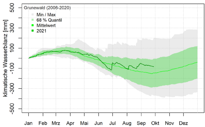
Klimaaufzeichnungen der Level II Freilandstation Grunewald (1101) der Jahre 2020 bis September 2021 für die mittlere Lufttemperatur (oben), die monatliche Niederschlagssumme (Mitte) und die klimatische Wasserbilanz als Differenz von Niederschlag und FAO-56 Gras-Referenzverdunstung (unten)
